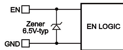
Figure 3: 6.5V-typ Zener Diode
